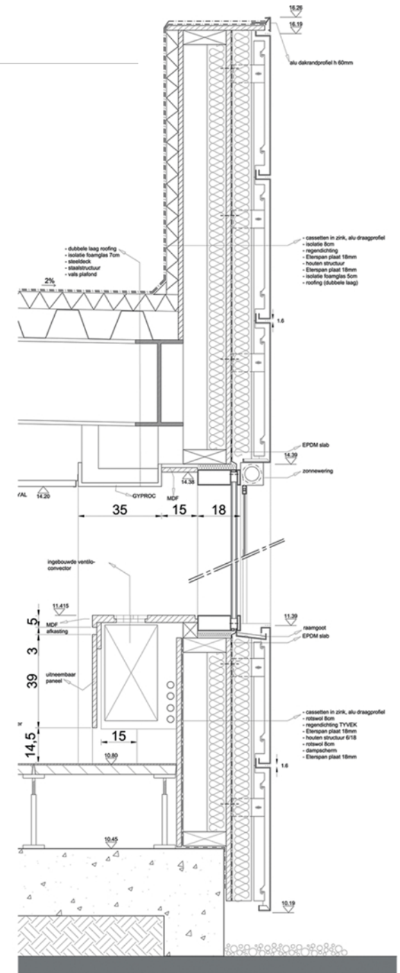
DETAIL ACHTERGEVEL
