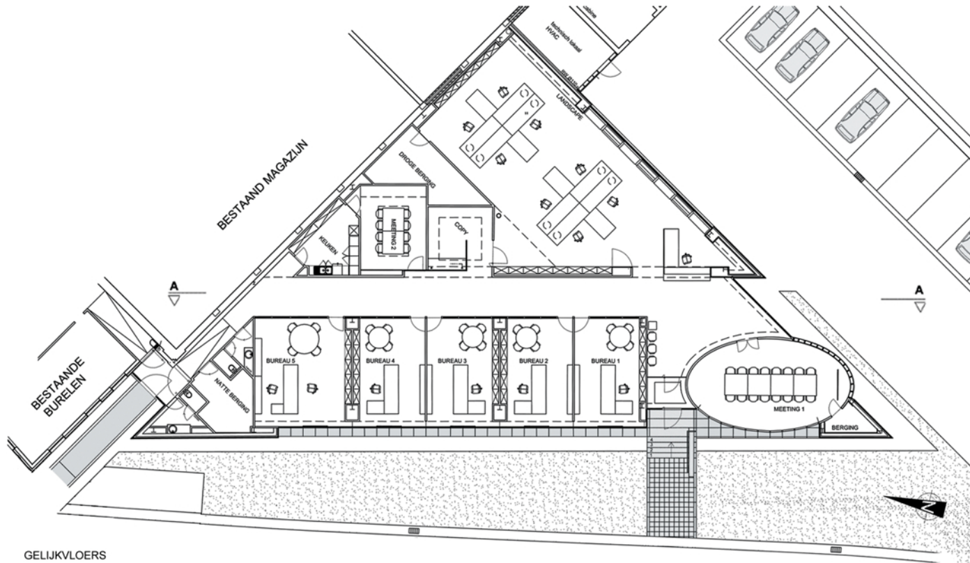
GELIJKVLOERS
